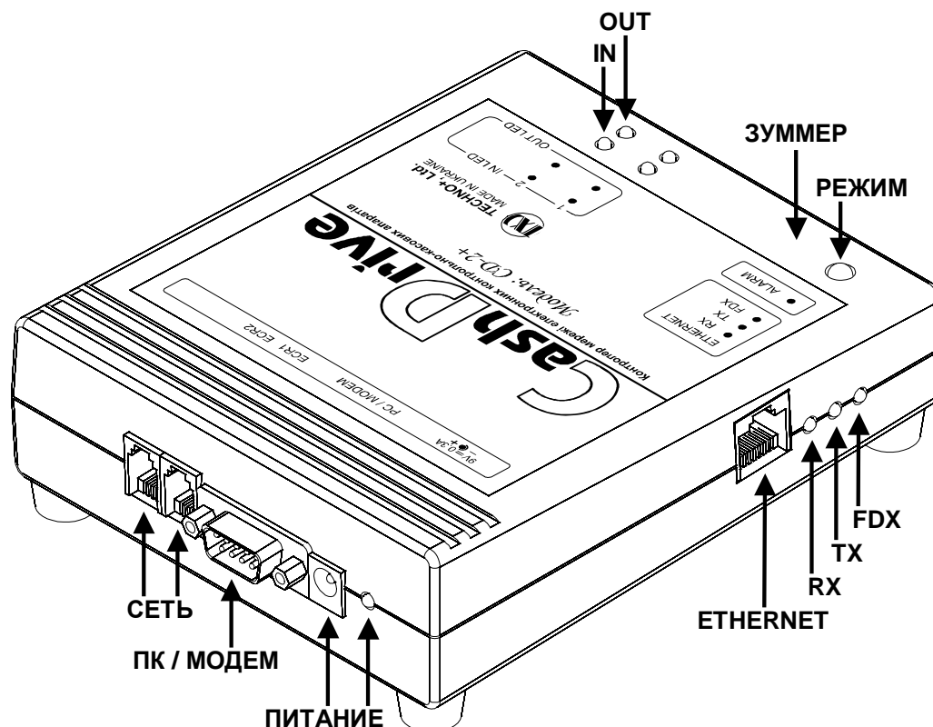
Рисунок 1 Контроллер «CashDrive CD-2+»
