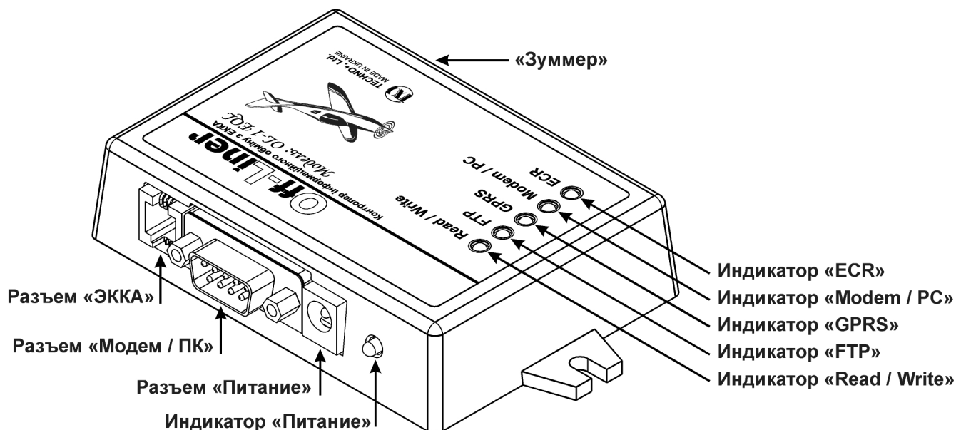
Рисунок 1 Контроллер «Off-Liner»
